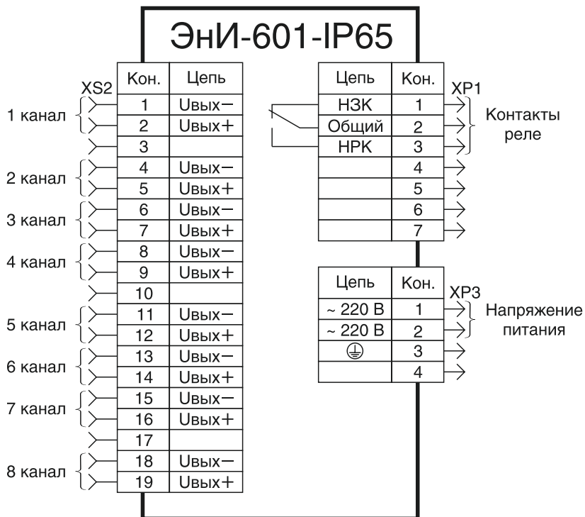
Рисунок Б.1 — Схема подключения БПП в исполнении IP65 (8 каналов)
